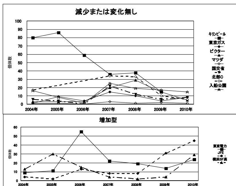
図4 シオカラトンボの調査地点別捕獲個体数の動向 上が減少傾向7地点、下が増加型3地点
