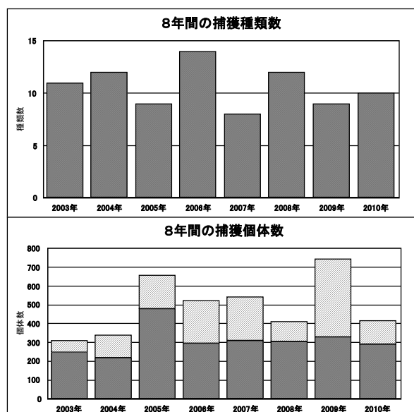
図1 8年間の捕獲種数（上）と個体数（下） 斜線はウスバキトンボ個体数を示す。
