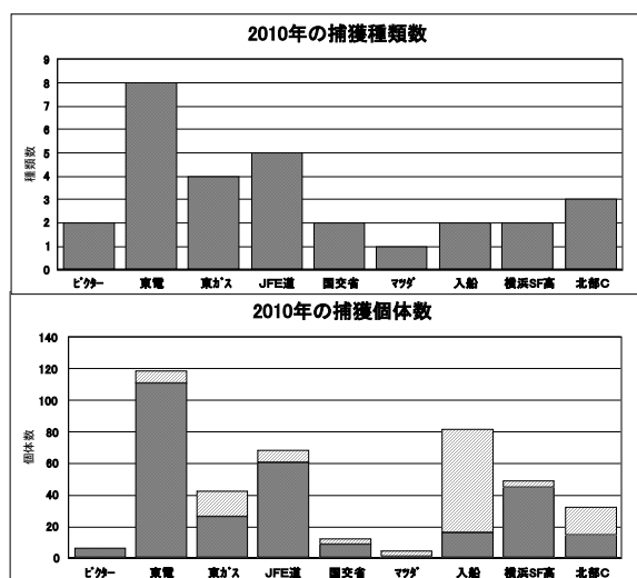
図2 2010年の調査地点別捕獲種数（上）と個体数（下） 斜線はウスバキトンボ個体数を示す。
